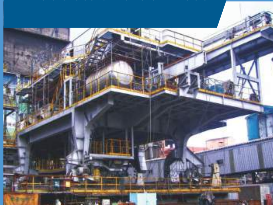
中龍推焦車 DSC coke oven pushing car
