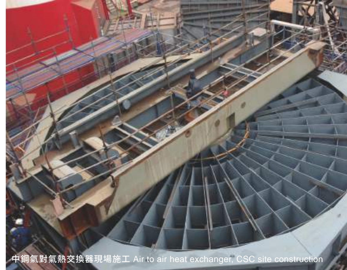
中龍 CDQ DSC CDQ
